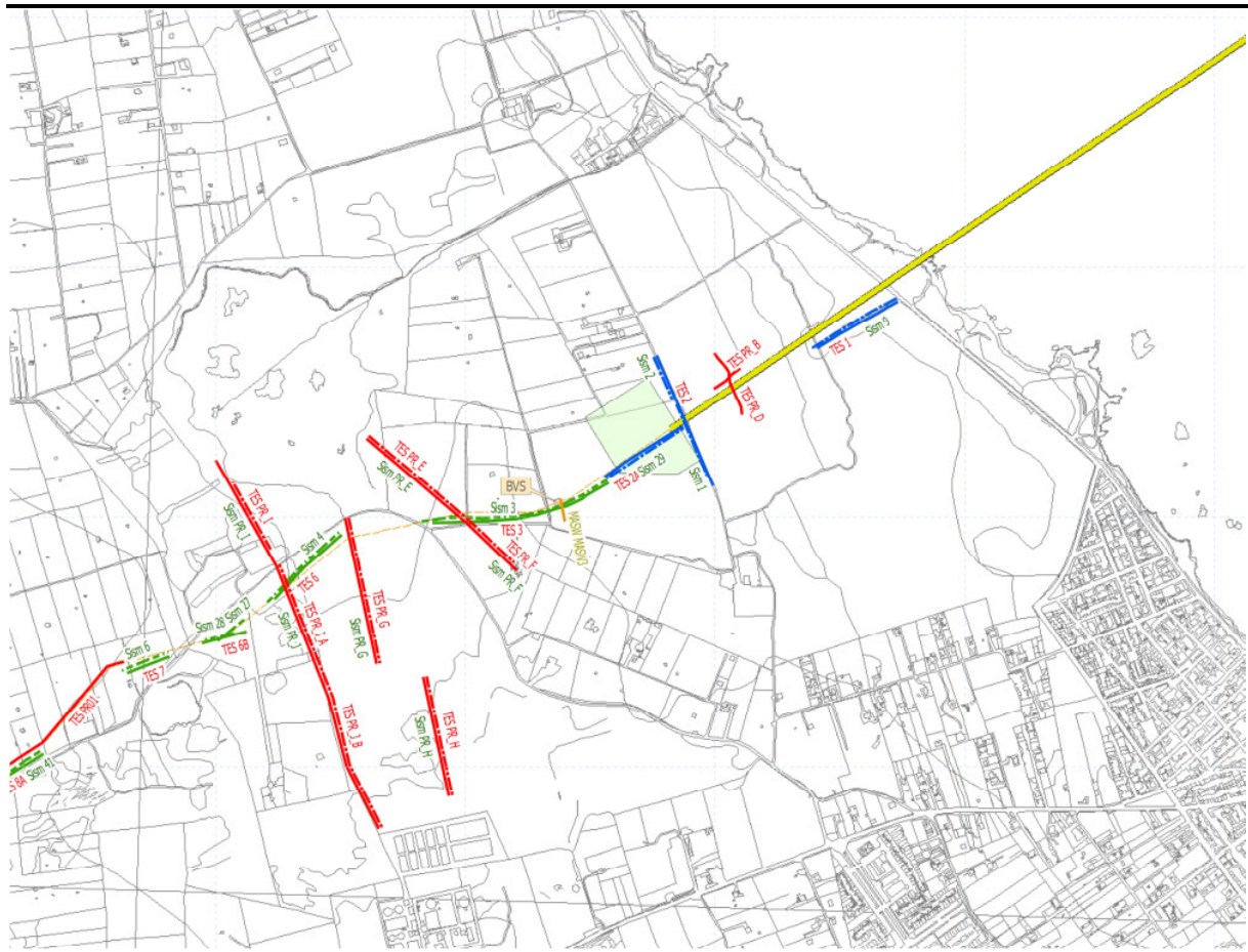
Figura 2.1 Ubicazione indagini geofisiche nell'area di approdo
