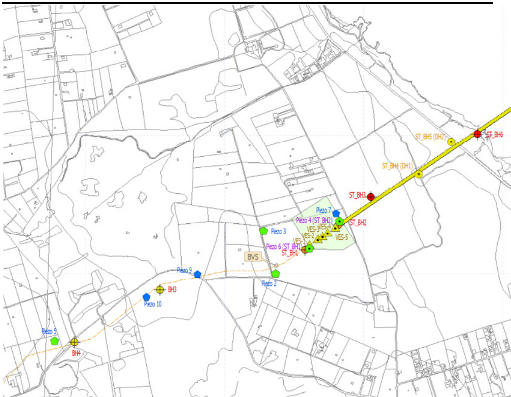
Figura 2.2 Ubicazione sondaggi geognostici e piezometri nell'area di approdo
