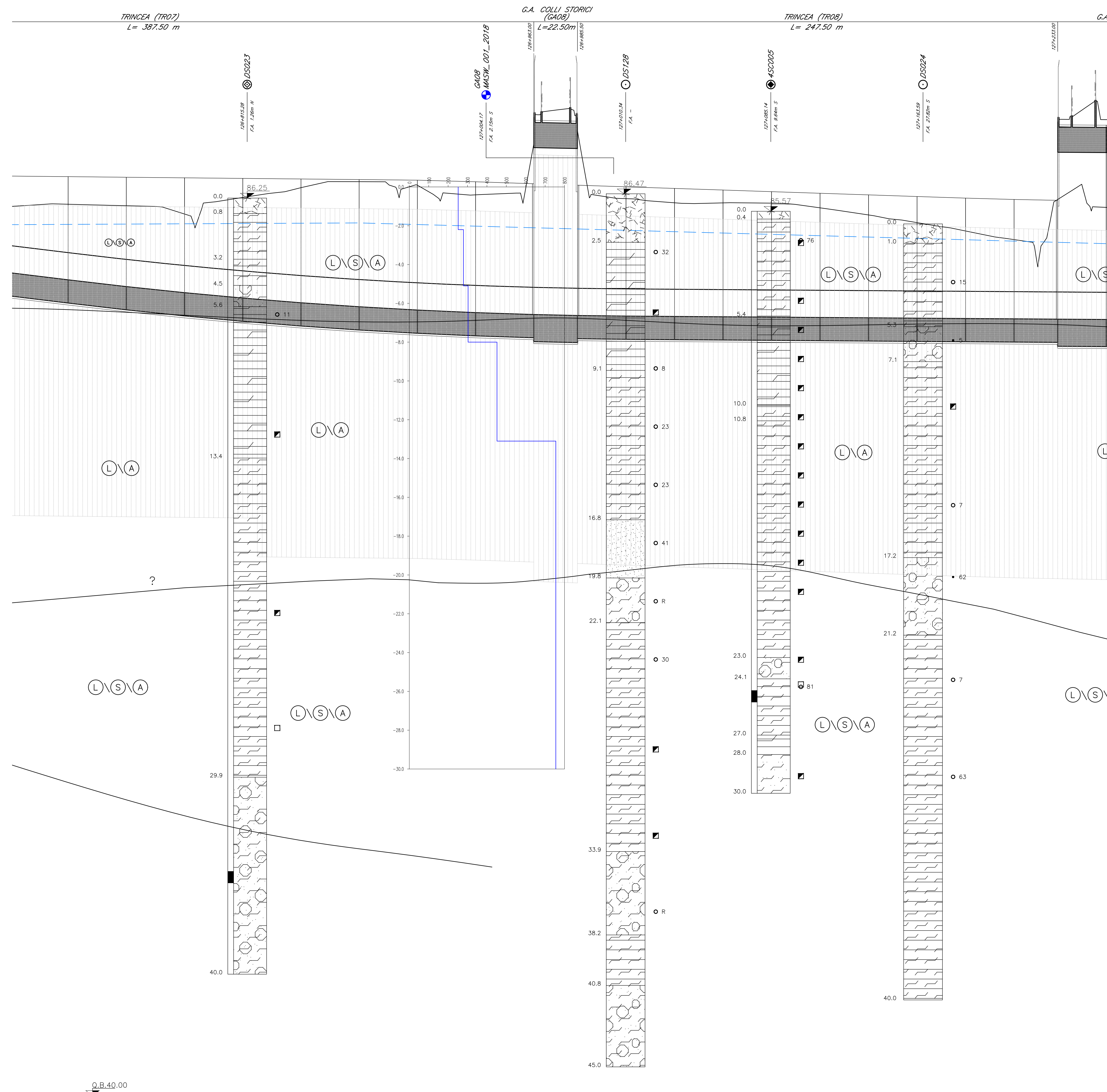
PROFILO STRATIGRAFICO SCALA 1:1000/1:100
