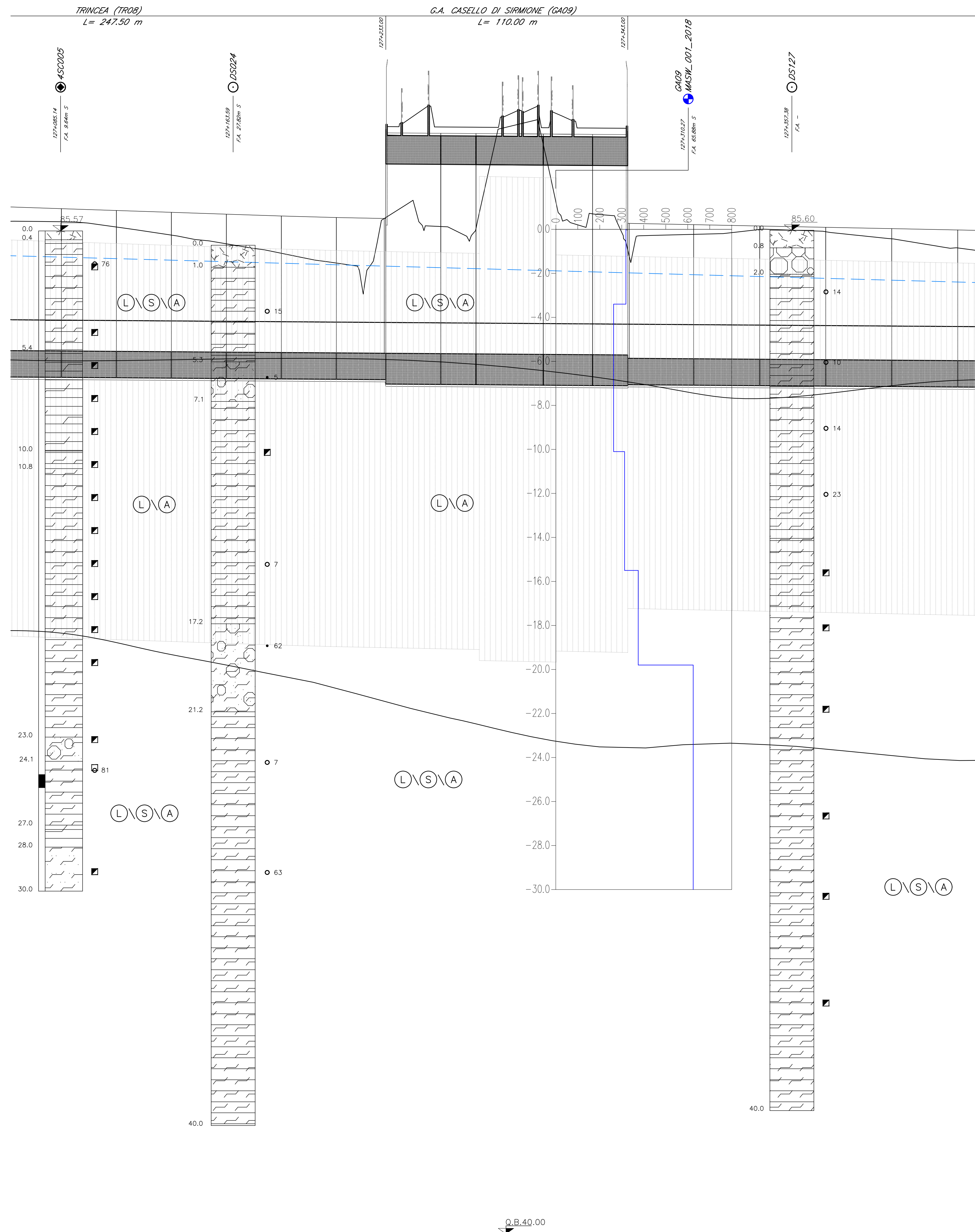
PROFILO STRATIGRAFICO SCALA 1:1000/1:100
