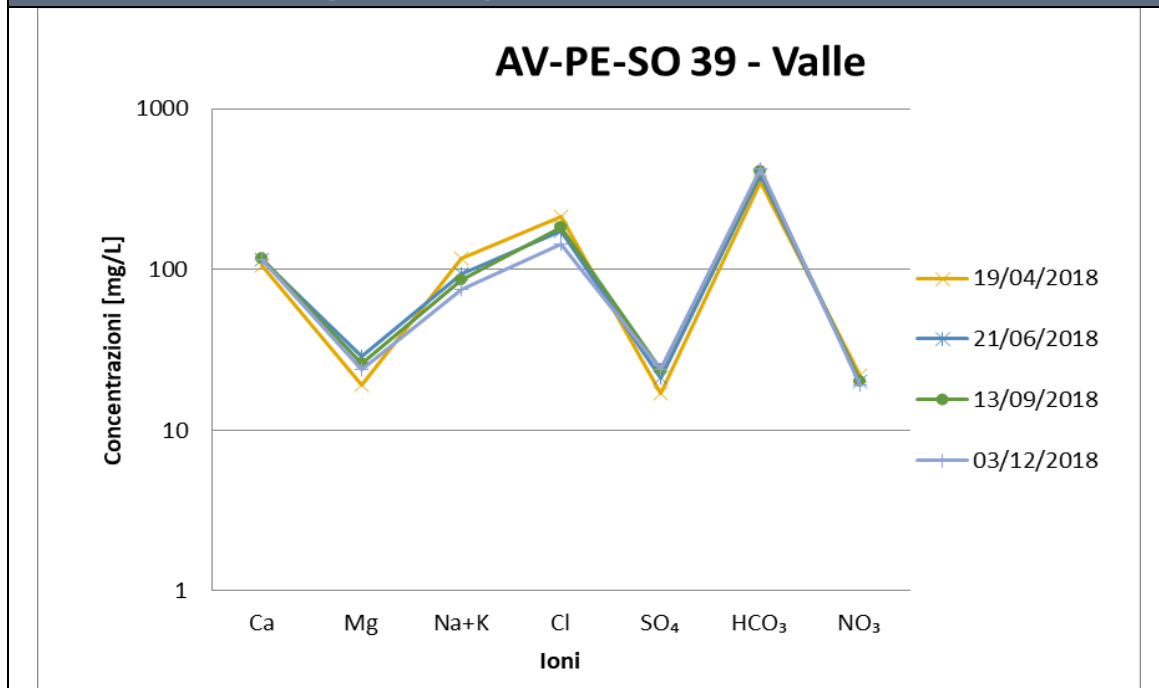
Figura 3-30 - Diagramma di Schoeller - AV-PE-SO-39
