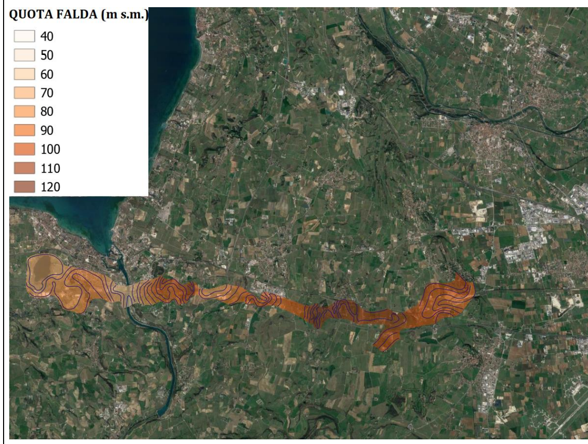
Figura 1-5 – Andamento delle Falde Sospese dell’Anfiteatro Morenico del Garda-Settore Veneto
