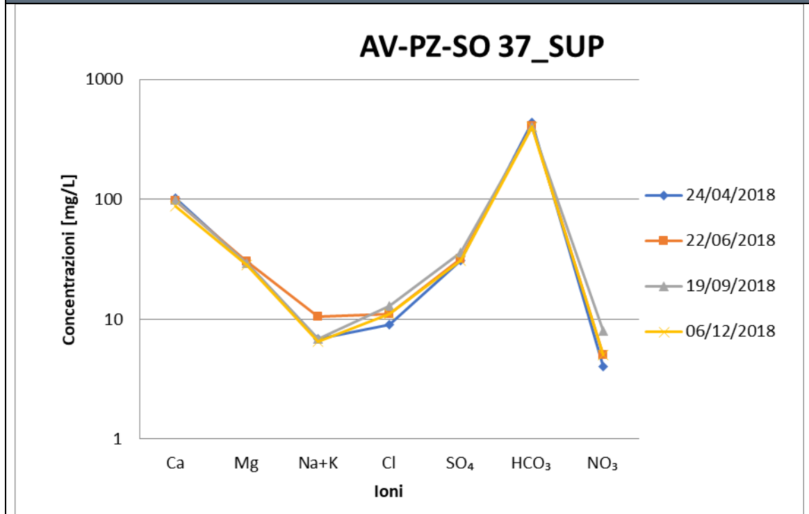
Figura 3-26 - Diagramma di Schoeller - AV-PZ-SO-37_SUP
