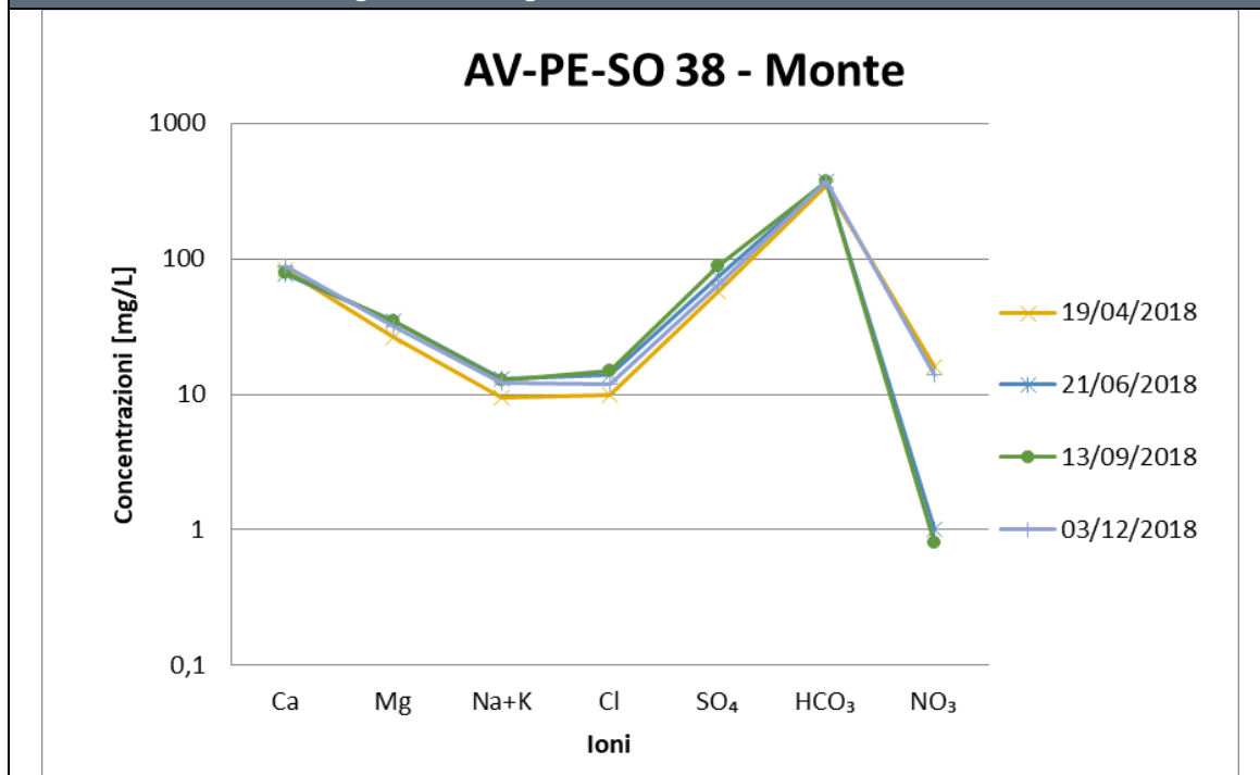
Figura 3-29 - Diagramma di Schoeller - AV-PE-SO-38
