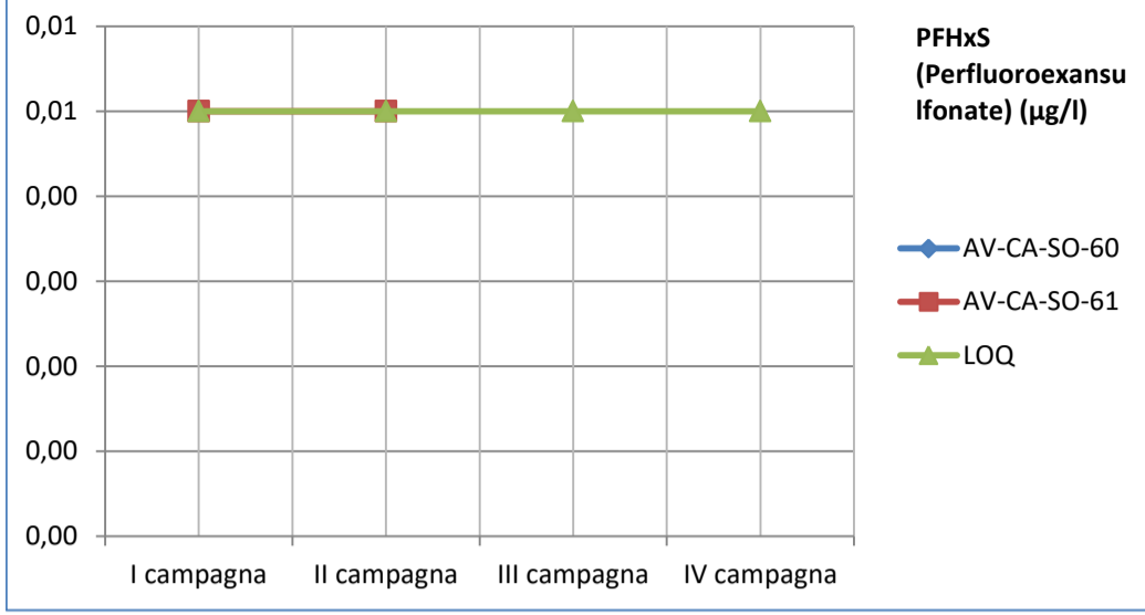
AV-CA-SO-60 (monte) - AV-CA-SO-61 (valle)
