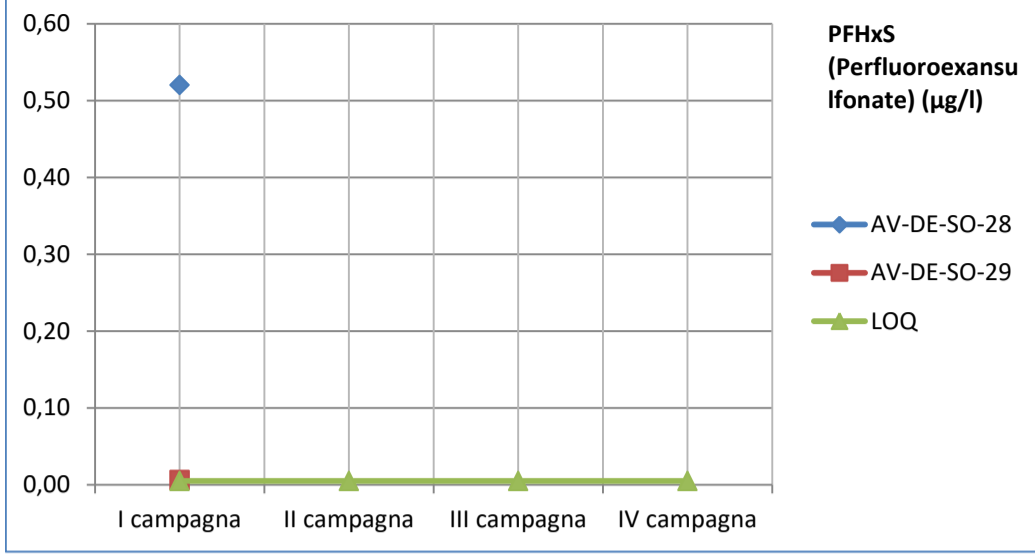
AV-DE-SO-28 (monte) - AV-DE-SO-29 (valle)
