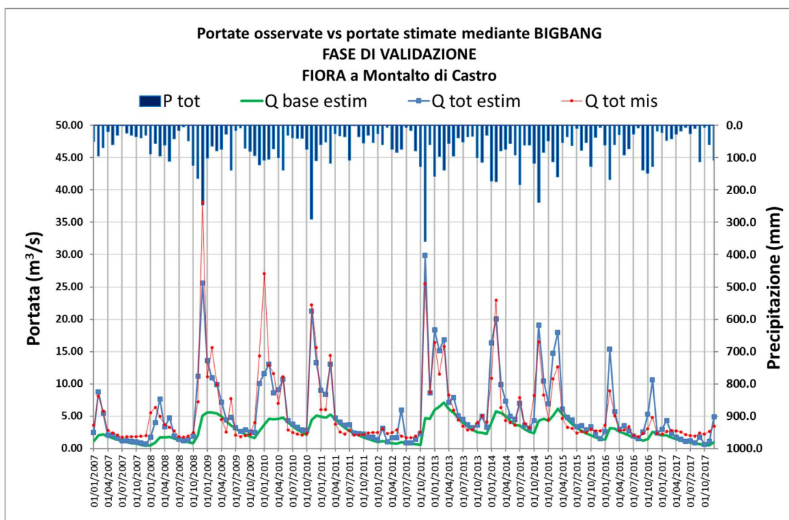
Figura 10.11 – Confronto tra le portate mensili misurate e stimate nella fase di validazione
